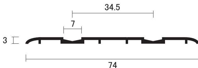
アルミ フロアーレール ダブル
