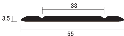
ウッド 二本引 フロアーレール 白木色
