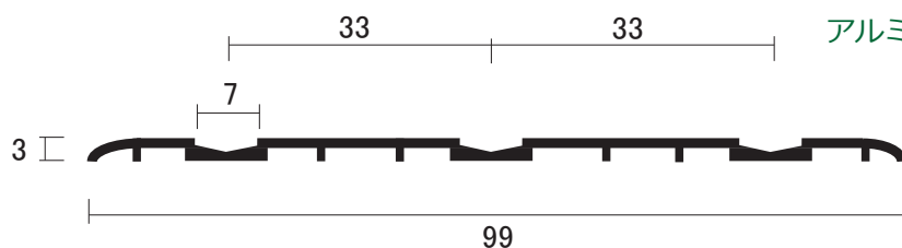
AL ラインレール シングル
