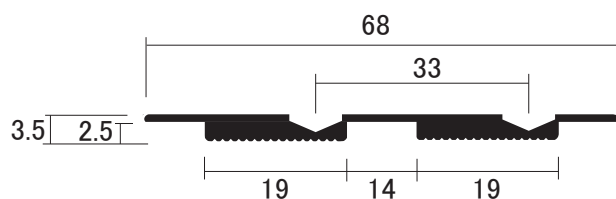
AL 敷居埋込みレール ダブル
