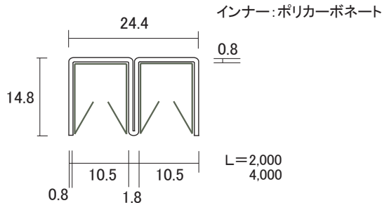
ステン 2号 直立下レール
