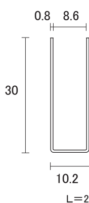
ステン 8mm ソロバン車用レール
