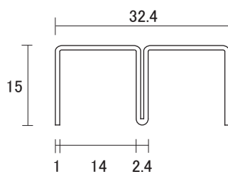
ステン 8mm ソロバン車用レール
