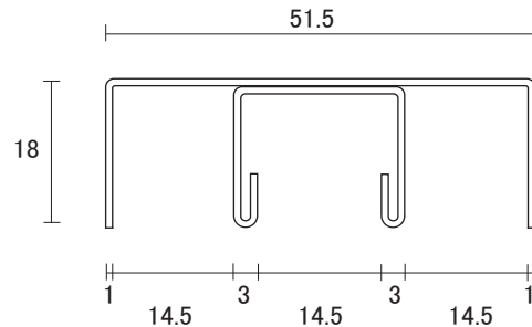
ステン 8mm 3線 堀込 上レール
