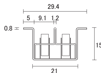
ステン ローラーレール
