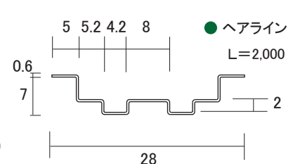
ステン 1号 直立下レール
