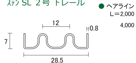
ステン SL 2号 下レール
