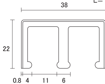
ステン S L 8mm 上レール
