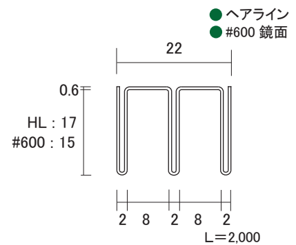
ステン 6mm 面打 上レール
