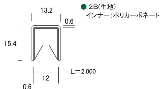
ステン 単線防虫上レール
