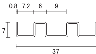
ステン 8mm ソロバン車用レール
