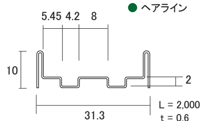
ステン 面付 直立下レール
