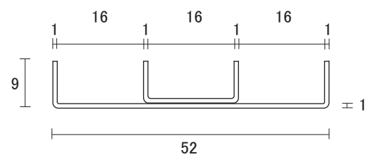
ステン 8mm 単線 上用 レール
