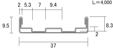
ステン SL 8mm 山型 レール
