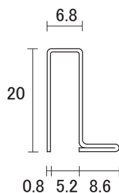
ステンレス 戸引手破損止 5mm用
