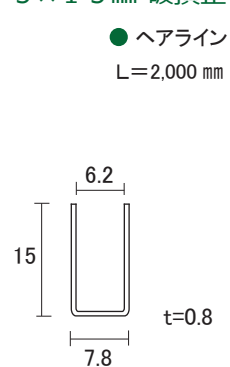
ステンレス 5×1 5mm 破損止
