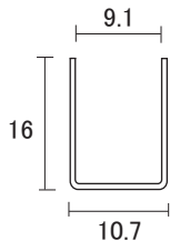
ステンレス 5mm 単線 ローラー用上レール
