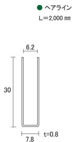
ステンレス 5×3 0mm 破損止
