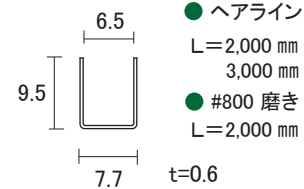
ステンレス 5mm 破損止
