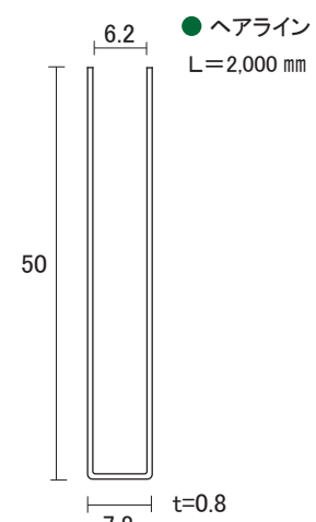
ステンレス 5×5 0mm 破損止
