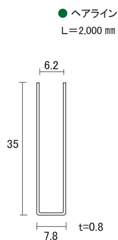
ステンレス 5×3 5mm 破損止
