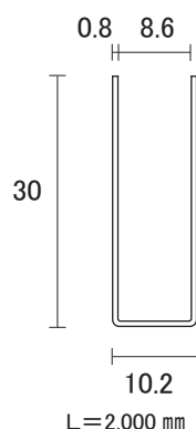
ステンレス 8×30mm コの字ハカマ ● ヘアライン
