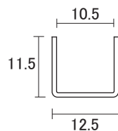
ステンレス 10-1 破損止
