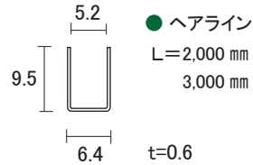
ステンレス 5mm - ② 破損止
