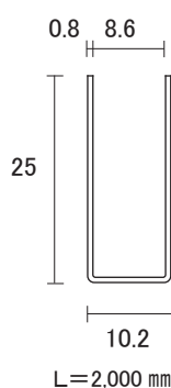
ステンレス 8×25mm コの字ハカマ ● ヘアライン
