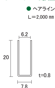
ステンレス 5×2 0mm 破損止
