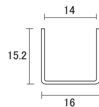
ステンレス 8mm 単線 上用 レール
