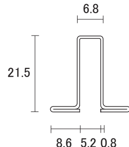
ステンレス 両 戸引手破損止 5mm用
