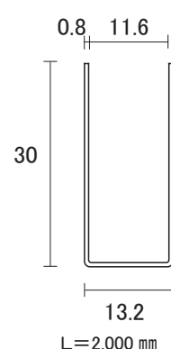
ステンレス 10×30mm コの字ハカマ ● ヘアライン
