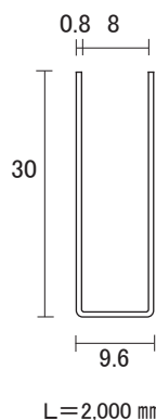
ステンレス 7×30mm コの字ハカマ ● ヘアライン
