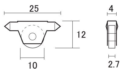
⑥ PB04 (真鍮ムク車)
