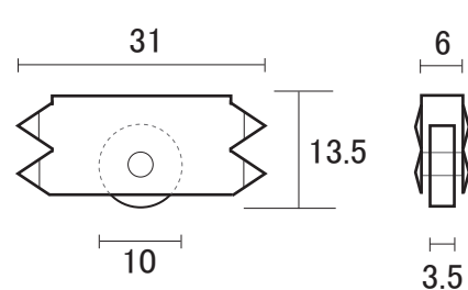
F-2019 (スチール車)
