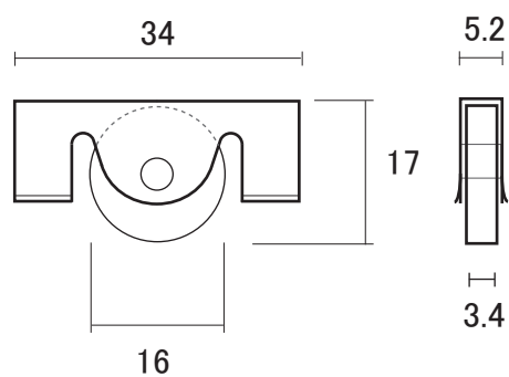
⑧ PBS33 (スチール車)
