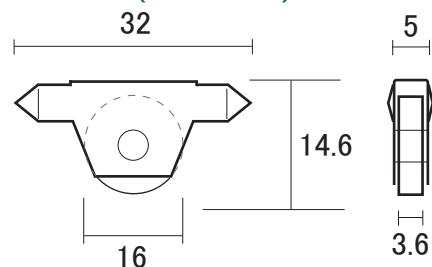
⑫PB30 (真鍮ムク車)
