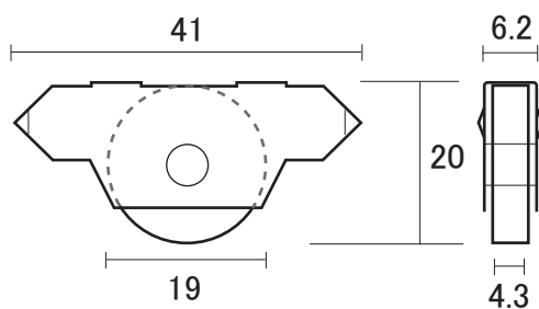
③ PB40 (スチール車)
