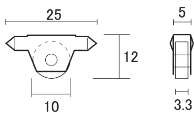
⑤ PB25 (真鍮ムク車)
