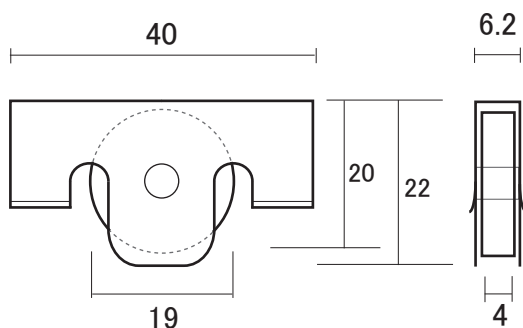
⑨PB40M / F-2017 (スチール車)
