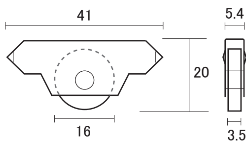
⑪PB38 (スチール車)
