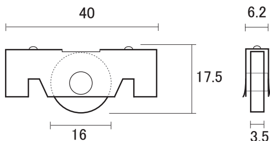
① AL 5 mmはかま用車 (スチール車)
