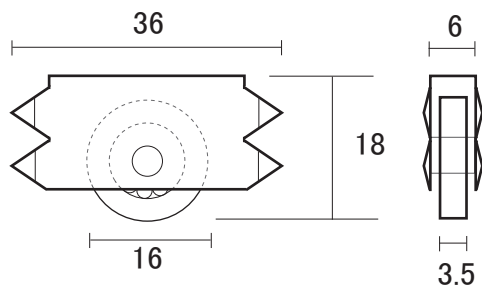
F-2028 (ジュラコン車)
