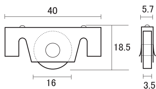
TIM-16 取付車 (スチール車)
