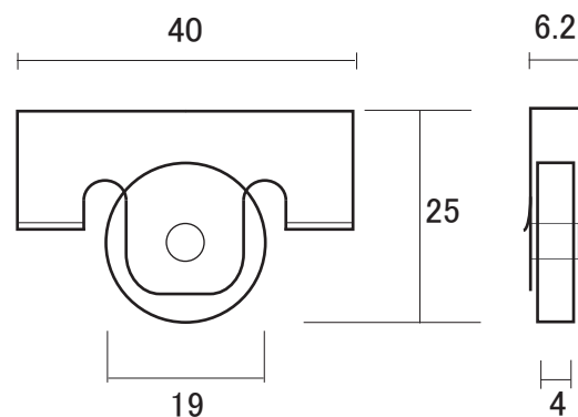
⑩PB40H / F-2016 (スチール車)
