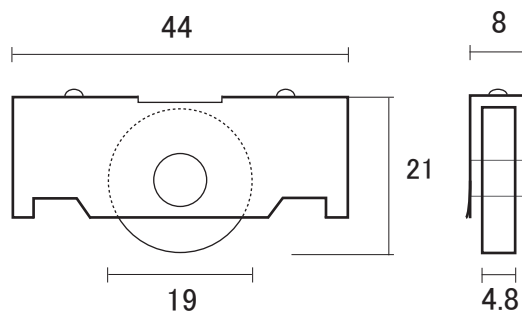
② AL 6 mmはかま用車 (スチール車)
