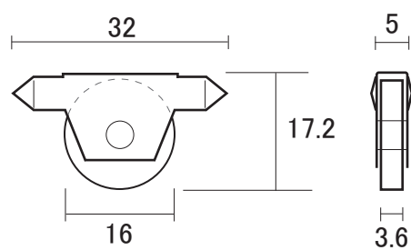
④ PB33 (スチール車)
