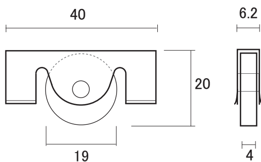
⑦ PBS40 (スチール車)
