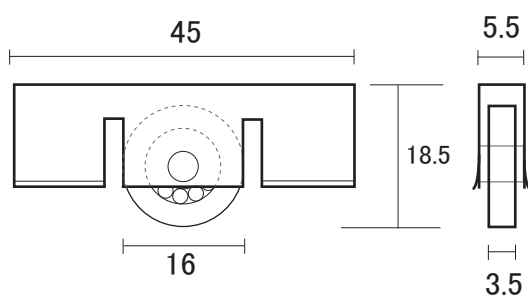
F-2027 (ジュラコン車)
