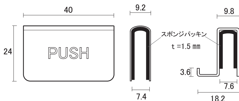
硝子用つまみ
