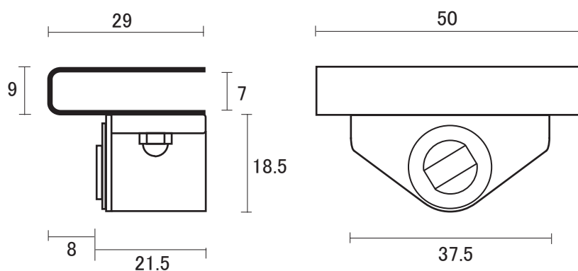
硝子天板用 マグネットキャッチ
