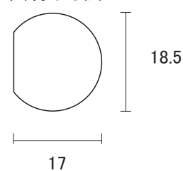
穴明け寸法
