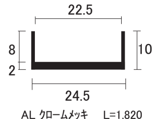
AL 戸当レール
