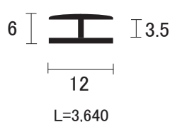
AL 端押ボーダー 12 mm用
