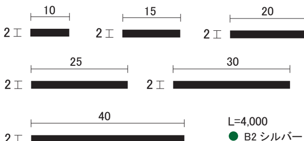
AL 平角棒 (フラットバー2mm厚)
