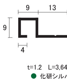
AL ミラーボーダー 9mm
