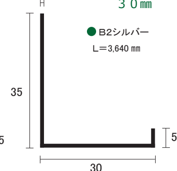
AL 看板ボーダー 30 mm
