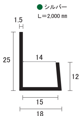
AL 端押ボーダー 12 mm用
