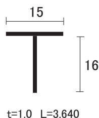
AL T(ティ) 字レール
