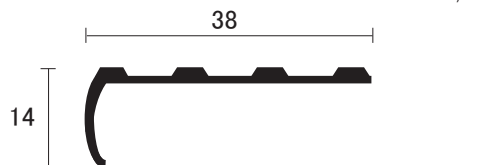
AL ノンスリップ
