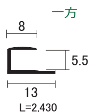
AL ジョイナー 5 mm
