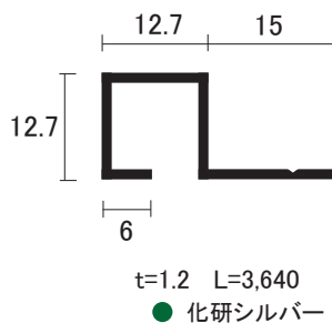
AL ミラーボーダー 12mm
