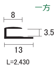
AL ジョイナー 3 mm
