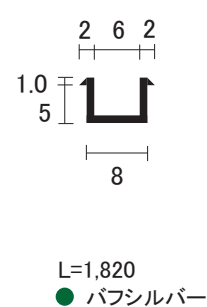
AL テーブルエッジ
