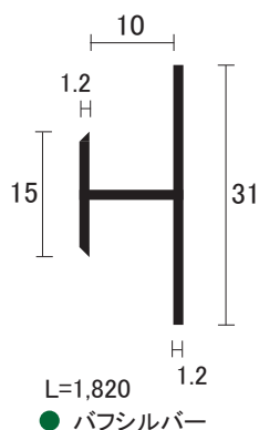
AL 鏡押 B-1
