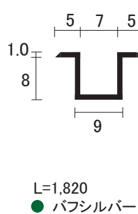
AL ミラーボーダー 12mm
