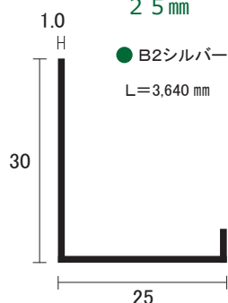
AL 看板ボーダー 25 mm
