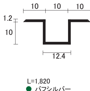
AL ミラーボーダー 12mm
