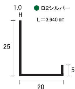
AL 看板ボーダー 20 mm
