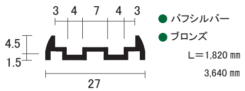
AL 65号5mm 面打 直立 下レール (5×40H ｽｶﾞ 専用)
