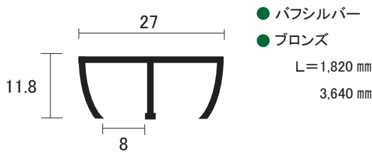
AL 5mm 面打 ｽｶﾞ用 上レール
