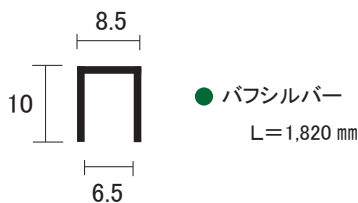
AL 5mm 単線 上レール
