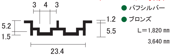
AL 55号5mm 堀込 直立 下レール (5×40H ｽｶﾞ 専用)
