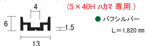
AL 直立 単線 下レール
