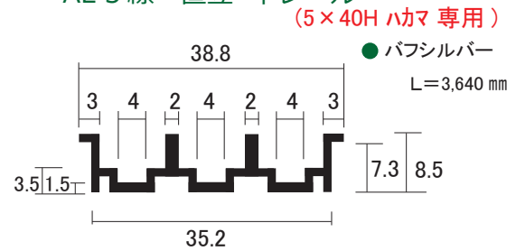
AL 3線 直立 下レール
