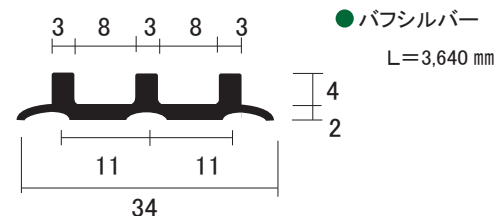
AL 3線 山型 レール
