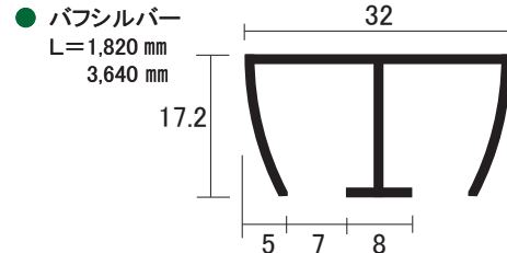
AL 70号 5mm 面打 直立 上レール
