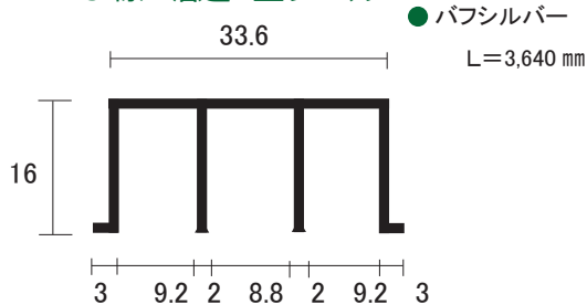
AL 3線 堀込 上レール
