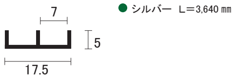
AL 5mm ジカ用 (車ナシ用) 下レール
