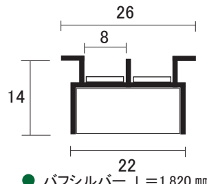
AL S Lローラーレール
