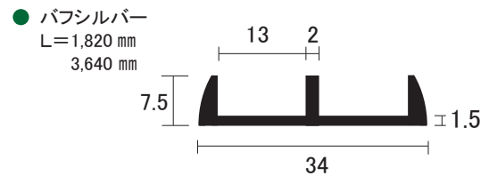
AL 70号 5mm 面打 直立 下レール
