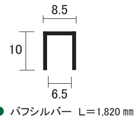
AL 5mm 単線 上レール
