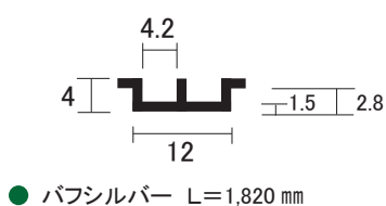
AL 3mm 家具用 堀込 下レール
