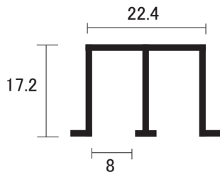
AL A-1型 上レール (7×40Hハカマ専用)
