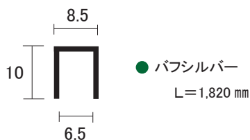
AL 6mm 単線 下レール
