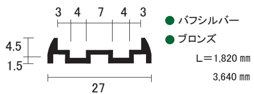
AL 65号5mm 面打 直立 下レール (5×40H ハカマ 専用)
