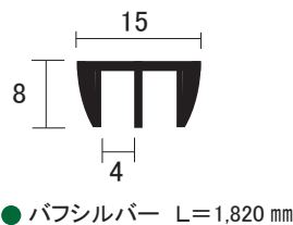
AL 3mm 面打 上レール
