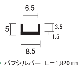
AL 5mm 単線 下レール
