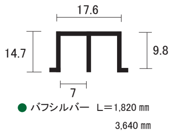
AL 5mm 家具用 堀込 上レール
