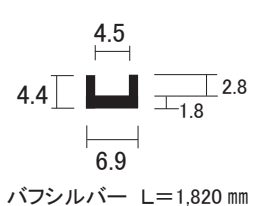
AL 3mm 単線 下レール
