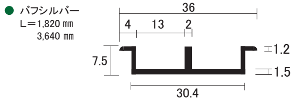
AL 戸当 レール
