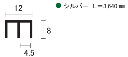
AL 3mm ジカ用 (車ナシ用) 上レール
