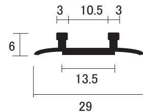
AL A-1型 山型 レール (7×40Hハカマ専用)
