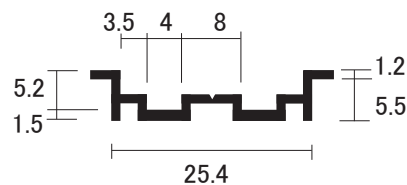
AL A-1型 堀込 直立下レール (7×40Hハカマ専用)
