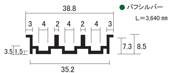
AL 3線 直立 下レール (5×40H ハカマ 専用)
