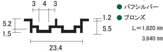
AL 55号5mm 堀込 直立 下レール (5×40H ハカマ 専用)
