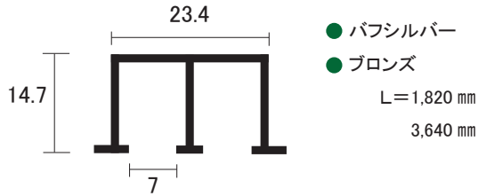
AL 55号5mm 堀込 直立 上レール
