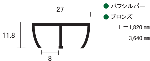
AL 5mm 面打 ハカマ用 上レール
