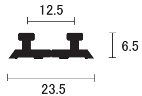
AL 6 mmはかま用 二列レール
