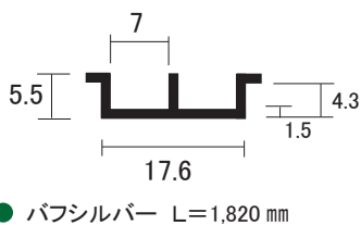
AL 5mm 家具用 堀込 下レール
