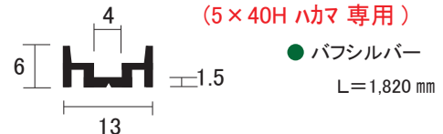
AL 直立 単線 下レール (5×40H ハカマ 専用)
