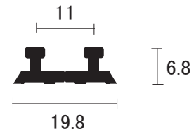
AL 5 mmはかま用 二列レール
