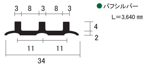
AL 直立 単線 下レール (5×40H ハカマ 専用)
