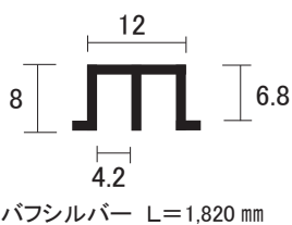
AL 3mm 家具用 堀込 上レール
