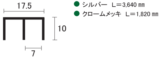
AL 5mm ジカ用 (車ナシ用) 上レール
