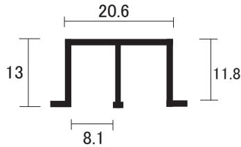
AL 5mm 堀込 上レール (ローラーレール用)
