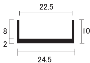
AL 戸当 レール
