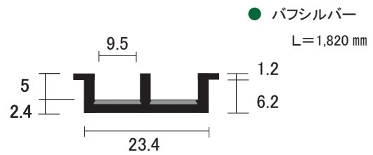
AL 5mm 山型 レール
