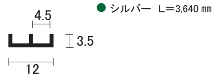
AL 3mm ジカ用 (車ナシ用) 下レール
