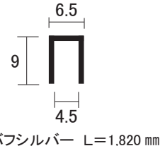
AL 3mm 単線 上レール
