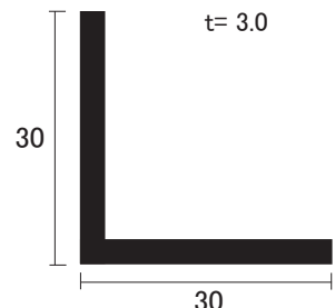
AL アングル 3 × 30 × 30
