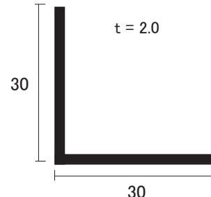
AL アングル 2 × 30 × 30
