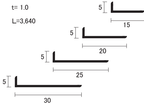
AL 不等辺アングル
