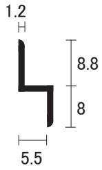
AL 5mm 一段アングル
