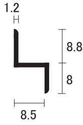
AL 8mm 一段アングル
