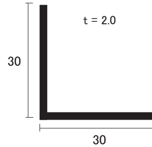
AL アングル 2 × 30 × 30
