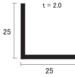
AL アングル 2 × 25 × 25
