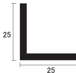
AL アングル 3 × 25 × 25
