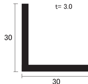
AL アングル 3 × 30 × 30
